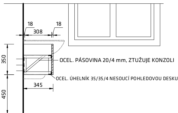
ŘEZ A - A', M1:25
