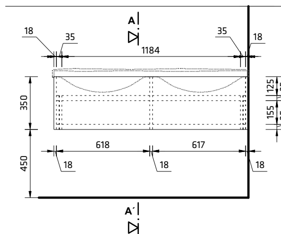
ČELNÍ POHLED, M1:25
