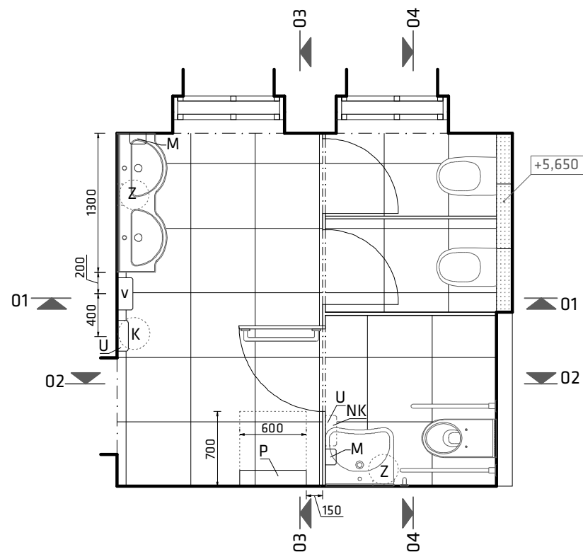
PŮDORYS WC ŽENY A VOZIČKÁŘI
